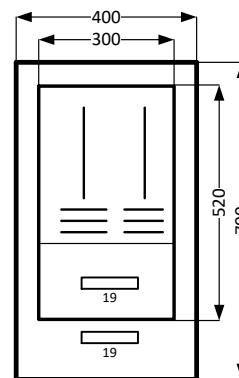
A 2.04 Wechselftafel 520 x 300 mm mit Schrank 700 x 400 x 225 mm
