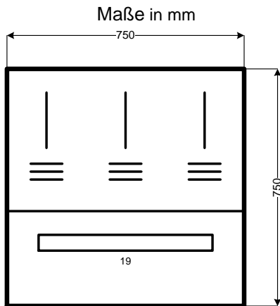
A 2.01 Wechselftafel 750 x 750 mm
